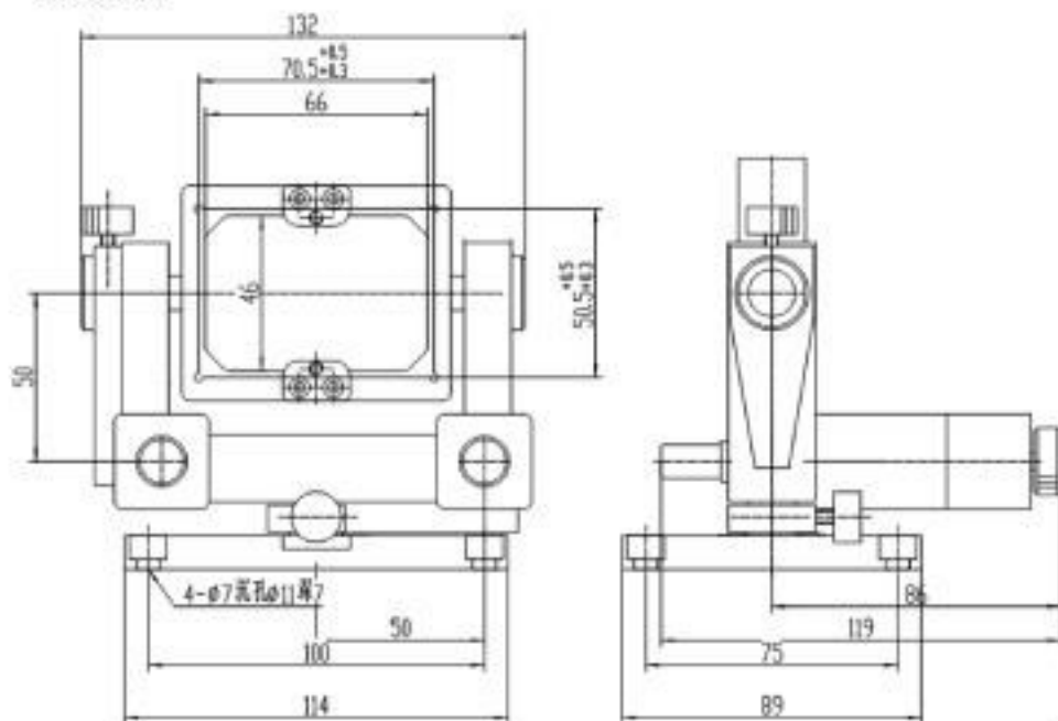
外形尺寸图
